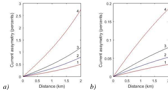
Рис. 3. Залежність коефіцієнта асиметрії РЛ за струмом від відстані до ЕРС для коефіцієнту поздовжньої асиметрії (у процентах) 1 (1), 2 (2), 3 (3), 7 (4), при опорі ізоляції рейки 1 Ом/км (а), 50 Ом/км (б) і при нульовій поперечній асиметрії.
