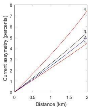
Рис. 5. Залежність коефіцієнта асиметрії РЛ за струмом від відстані до ЕРС для коефіцієнту поздовжньої асиметрії (у процентах) 1 (1), 2 (2), 3 (3), 7 (4) при опорі ізоляції рейки 1 Ом/км і коефіцієнту поперечної асиметрії 5 %.
