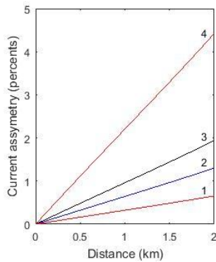
Рис. 4. Залежність коефіцієнта асиметрії РЛ за струмом від відстані до ЕРС для коефіцієнту поперечної асиметрії (у процентах) 1 (1), 2 (2), 3 (3), 7 (4) при опорі ізоляції рейки 1 Ом/км і при нульовій поздовжній асиметрії
