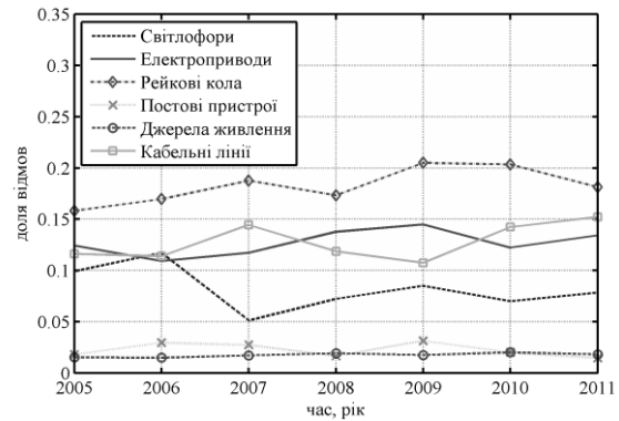
Рис. 1. Часова залежність частоти відмов об'єктів ЕЦ
