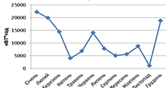
Рис.1 Графік спожитої електроенергії на власні потреби підстанції, кВт·год
