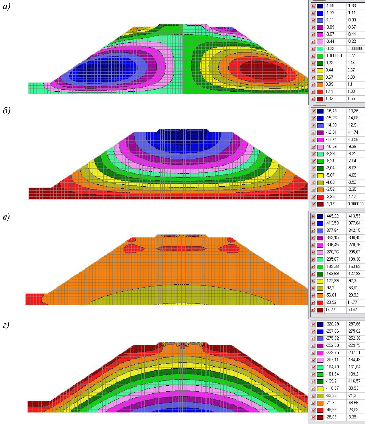
Рис. 5. Ізолінії та ізополя переміщень та напружень у випадку насипу із однорідного матеріалу, 2-а схема завантаження: а) переміщення по осі X (горизонтальна); б) переміщення по осі Z (вертикальна); в) нормальні напруження по осі X (горизонтальна); г) нормальні напруження по осі Z (вертикальна)
