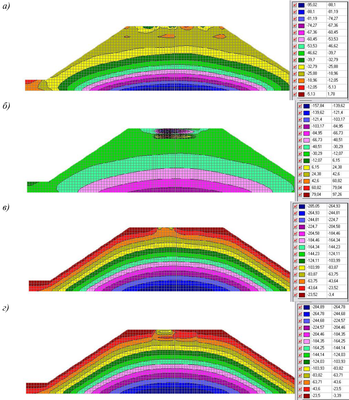
Рис. 7. Ізолінії та ізополя переміщень та напружень, 1-а схема завантаження: а) нормальні напруження по осі X (без підсилення геосинтетиками); б) нормальні напруження по осі X (з комбінованим підсиленням геосинтетиками); в) нормальні напруження по осі Z (без підсилення геосинтетиками); г) нормальні напруження по осі Z (з комбінованим підсиленням геосинтетиками)
